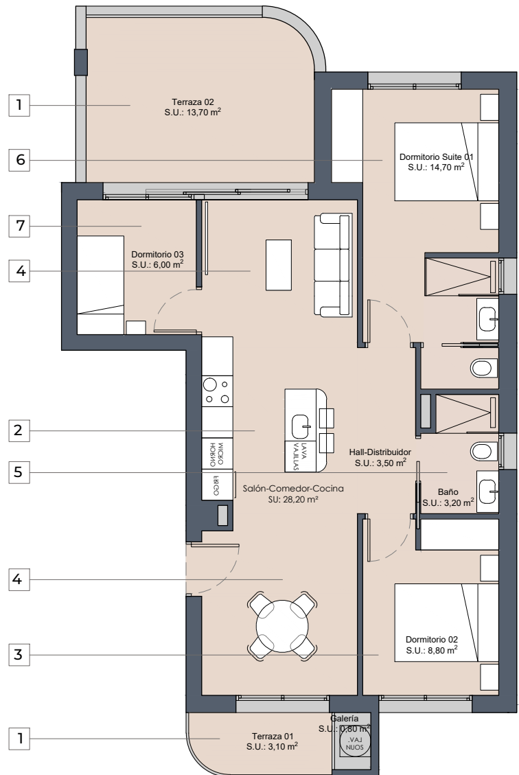
PLANTA PRIMERA
