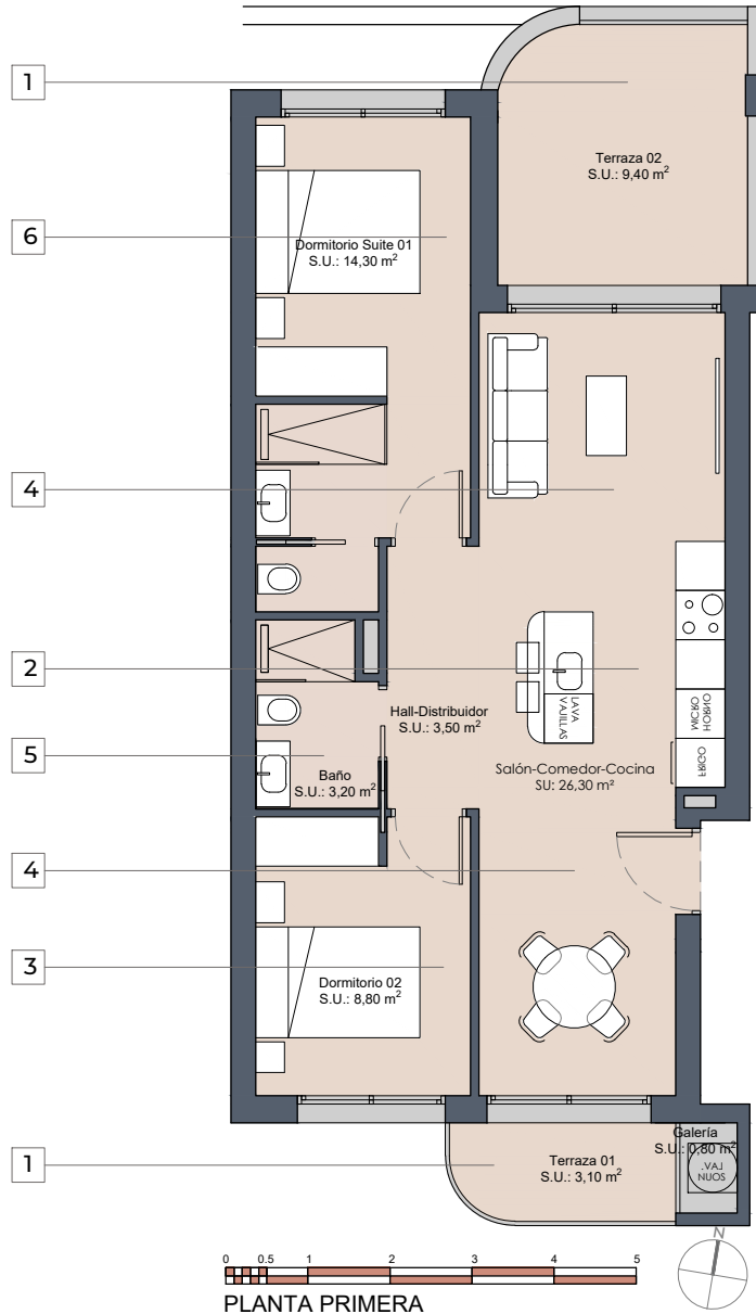
PLANTA PRIMERA
