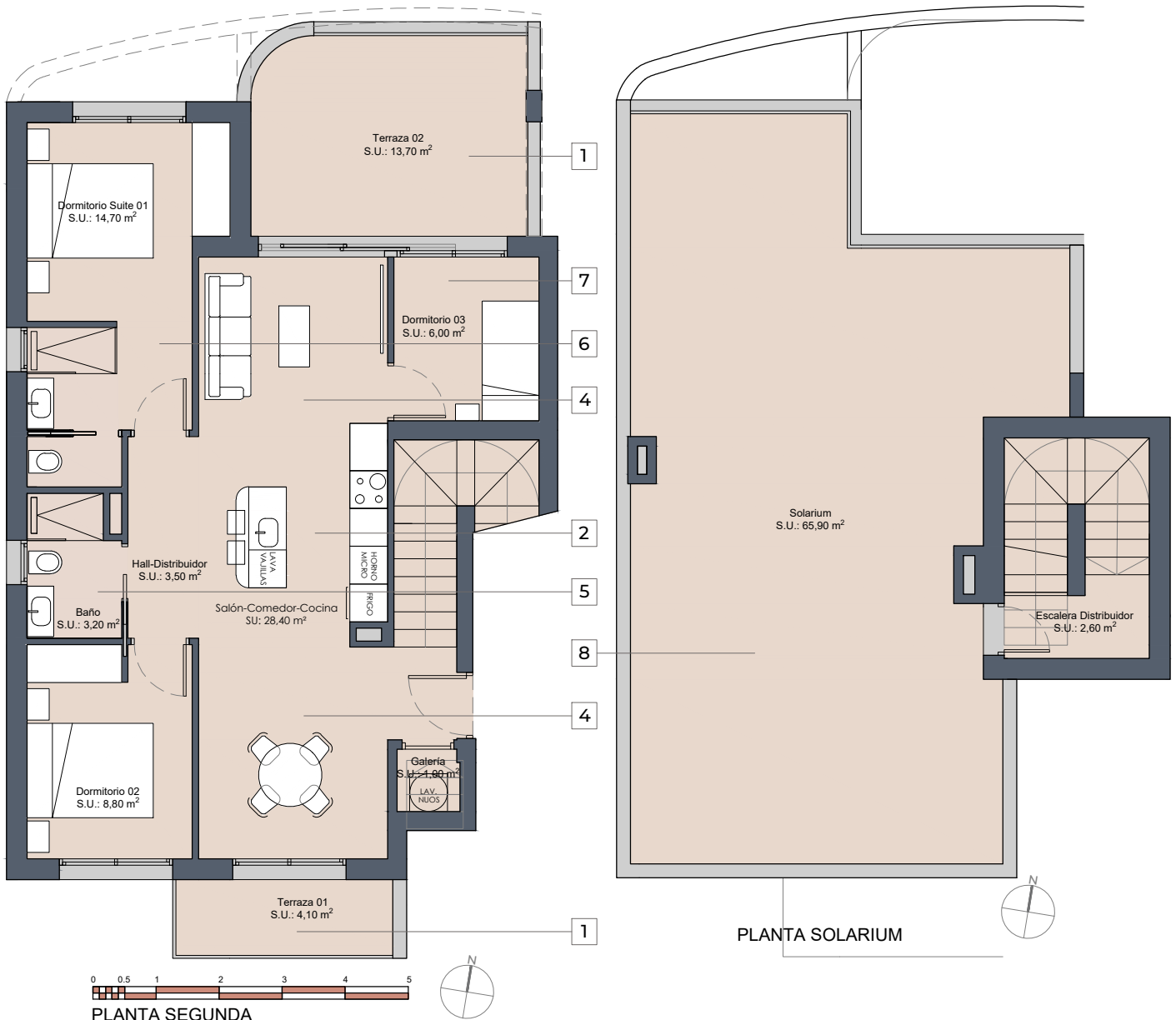
PLANTA SEGUNDA
